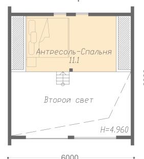
План антресоли
