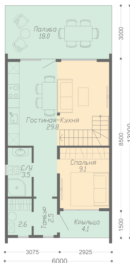
ПЛАН ПЕРВОГО ЭТАЖА
