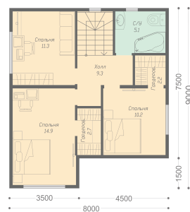
План второго этажа
