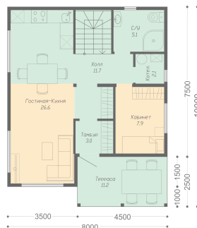
План первого этажа
